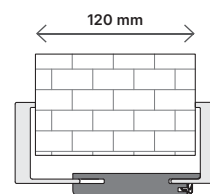
MAXIMÁLNÍ ROZSAH regulace bez zkrácení pera záklopu
