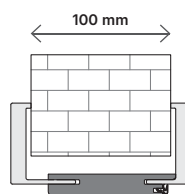
STANDARDNÍ ROZSAH regulace bez zkrácení pera záklopu
