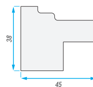
PROFIL LIŠTY
