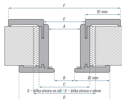
Rozměry reverzní zárubně (mm) / Rozměry reverznej zárubne (mm)
