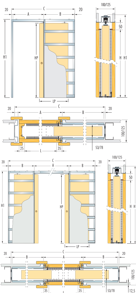
Tabulka rozměrů pro jednokřídlé provedení Tabulka rozmerov pre jednokřídlé prevedenie
