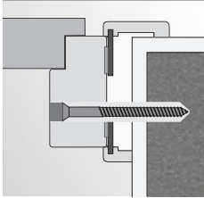
montáž pěnou a kotvy do zdivné stěny
