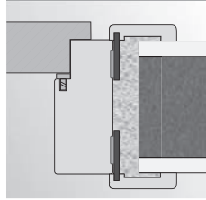
montáž pěnou ve zdivné stěně
