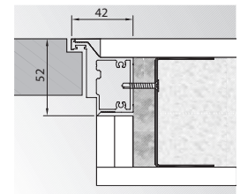
Reverzní polodrážka (otevřené dovnitř)
