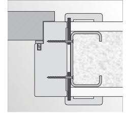
montáž pomocí šroubů do stěny SDK
