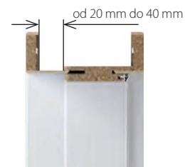
zárubeň s širokým perem volitelně za příplatek
