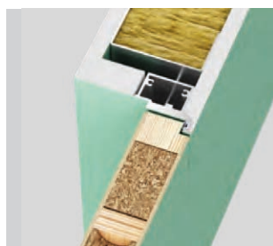
Reverzní falc (otvírání dovnitř) - levé dveře
