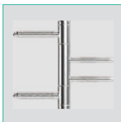
třídní závěsy do zár. PORTA System - technická rozteč
