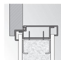
zároveň Rohová VELKÁ montáž na stěně SDK
